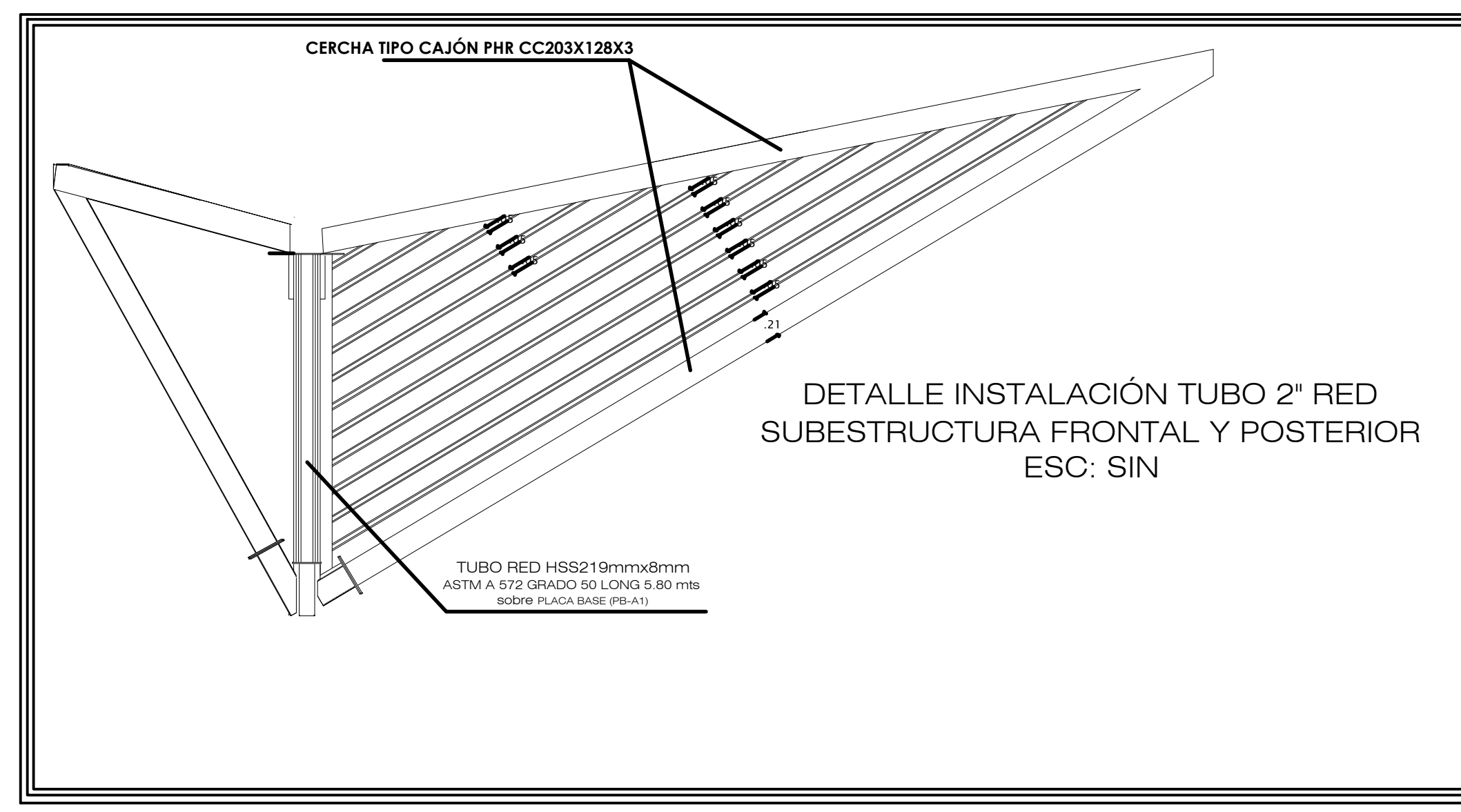
DETALLE TUBO RED 2\"/>
